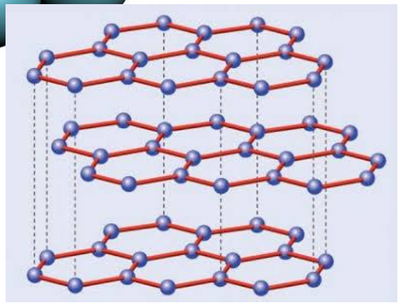
Estructura cúbica
